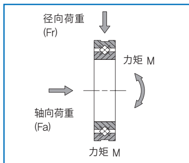
图4. 轴承载荷
